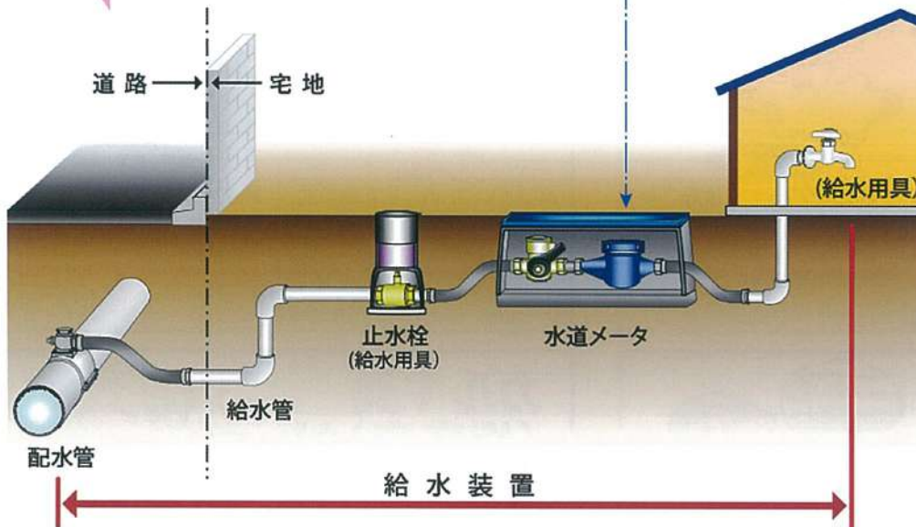
図-1 給水装置の概念図 (1)
